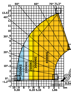
Manitou 1440
