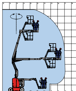
Manitou 120 AETJ
