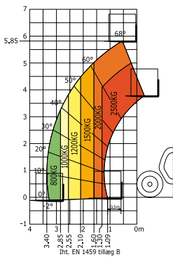
Manitou 625
