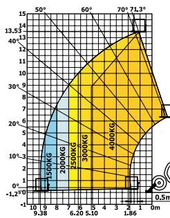
Manitou 1440
