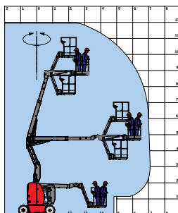
Manitou 120 AETJ
