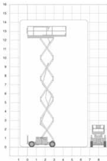
Genie GS4069RT
