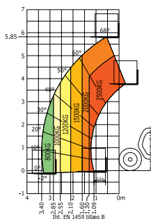
Manitou 625
